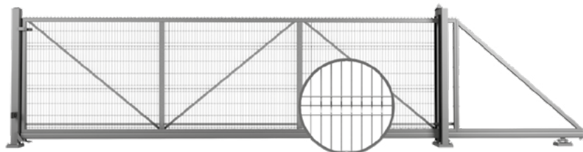
Skydeport med fyldning af VEGA B-trådnetspaneler, som er skruet fast i konstruktionen – vist fra den indhegnede side.
