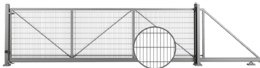
Skydeport med fyldning af VEGA 2D Super-trådnetspaneler, som er skruet fast i konstruktionen – vist fra den indhegnede side.
