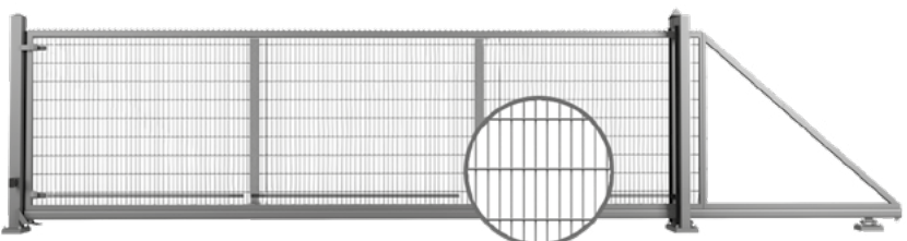
Skydeport med VEGA 2D Super-gitterpanelfyldning, som er svejset fast til konstruktionen – vist fra den indhegnede side.
