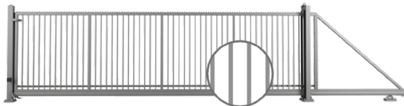
Skydeport med fyldning, der består af boksprofiler på 25 x 25 [mm], som er svejset fast i konstruktionen – vist fra den indhegnede side.
