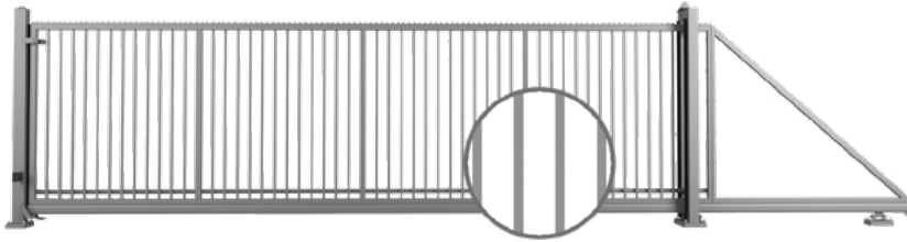
SKYDEPORT MED FYLDNING, DER BESTÅR AF BOKSPROFILER PÅ 25 X 25 [MM], SOM ER SVEJSET FAST I KONSTRUKTIONEN – VIST FRA DEN INDHEGNEDE SIDE.
